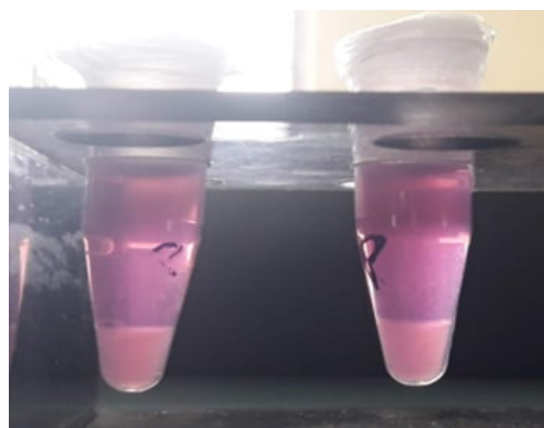
Fig. 3: Prodigiosin pigment
